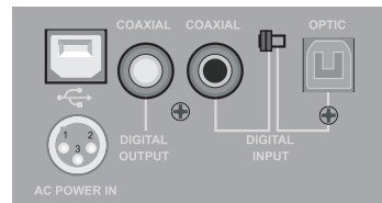
Fig. 2.6: Sección del panel trasero (con UD)
