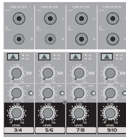
Fig. 2.2: Controles y conectores de los canales estéreo
