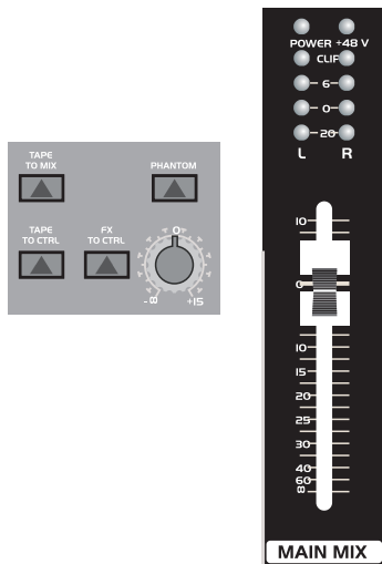
Fig. 2.4: Elementos de control de la sección principal.
