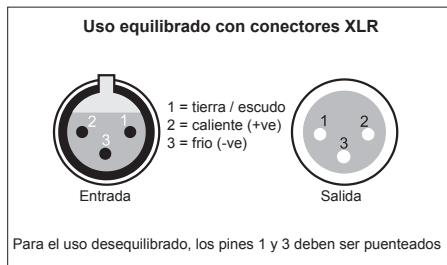
Fig. 4.1: Conexiones XLR
